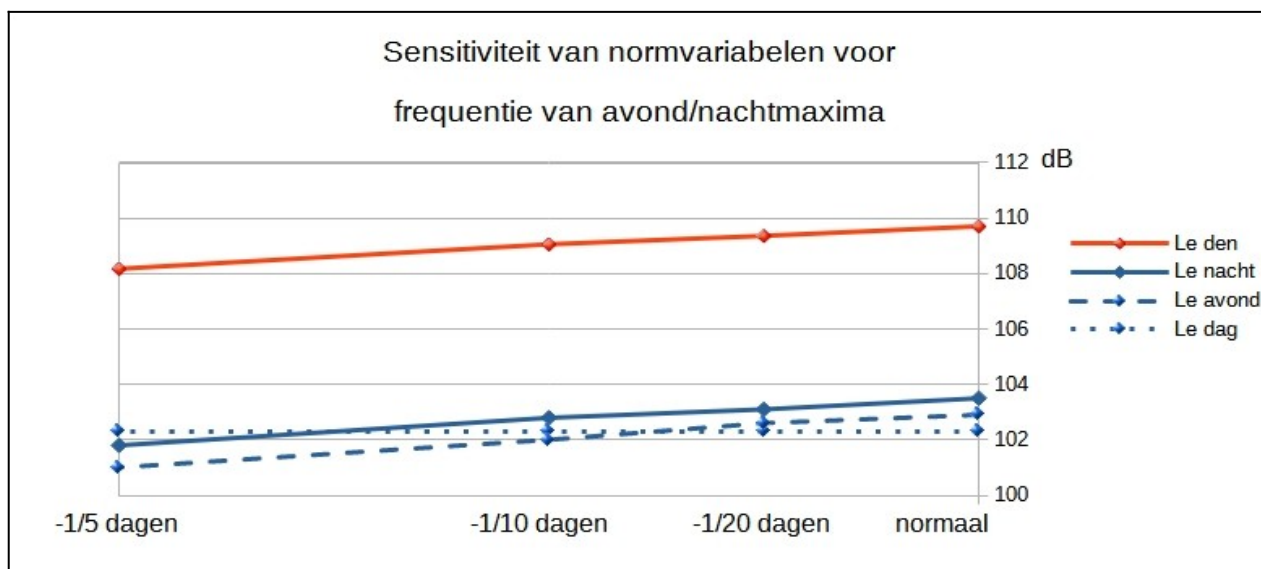
Figuur 11: Afname van de jaargemiddelde geluidsbelasting door het vervangen van het 12 uren avond/nacht windmaximum door windstilte eens per gemiddeld 5, 10, 20 dagen.
