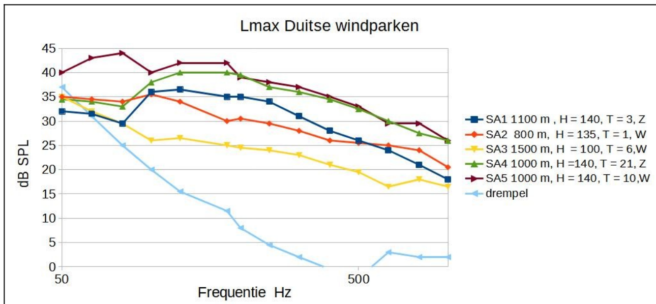
Figuur 8: H: ashoogte, T: aantal turbines, Z: zomer, W: winter; gehoordrempel ISO-28961-P10 Onderzoek Duitse overheid 34 : maximale geluidniveaus windparken SA1 – SA5
