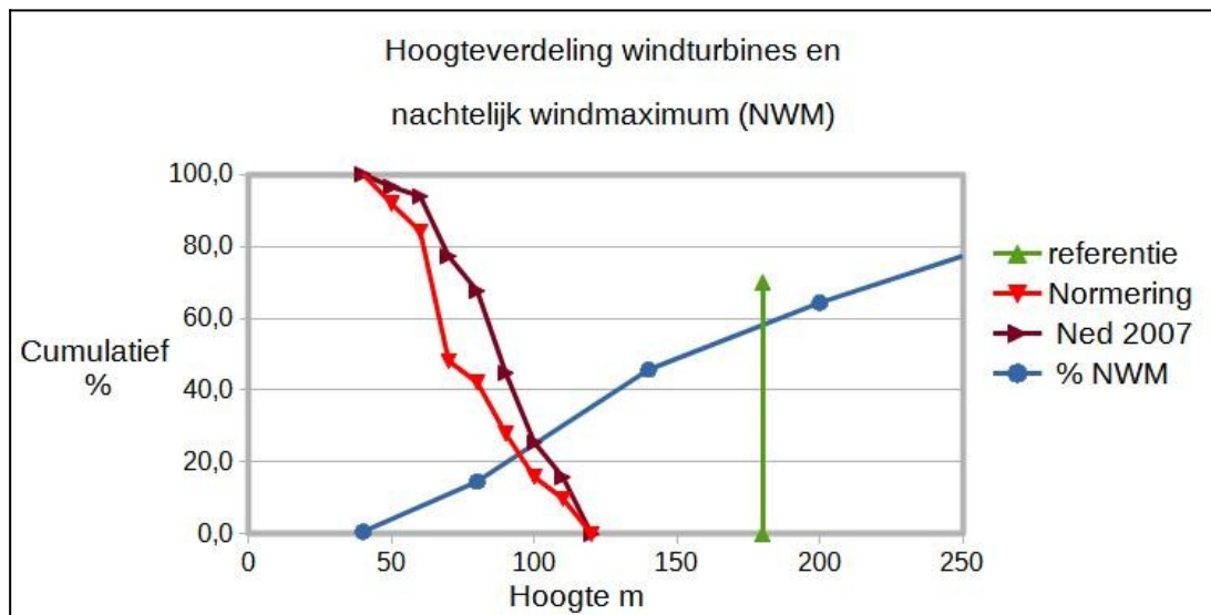
Figuur 3: Cumulatieve kans op nachtelijke windmaxima (NWM) en de ashoogteverdeling van windturbines uit het dosis-effectonderzoek Nederland 2007 en twee Zweedse onderzoeken (2000, 2005) die samen de basis vormen van de Nederlandse normering . 27,29,30
