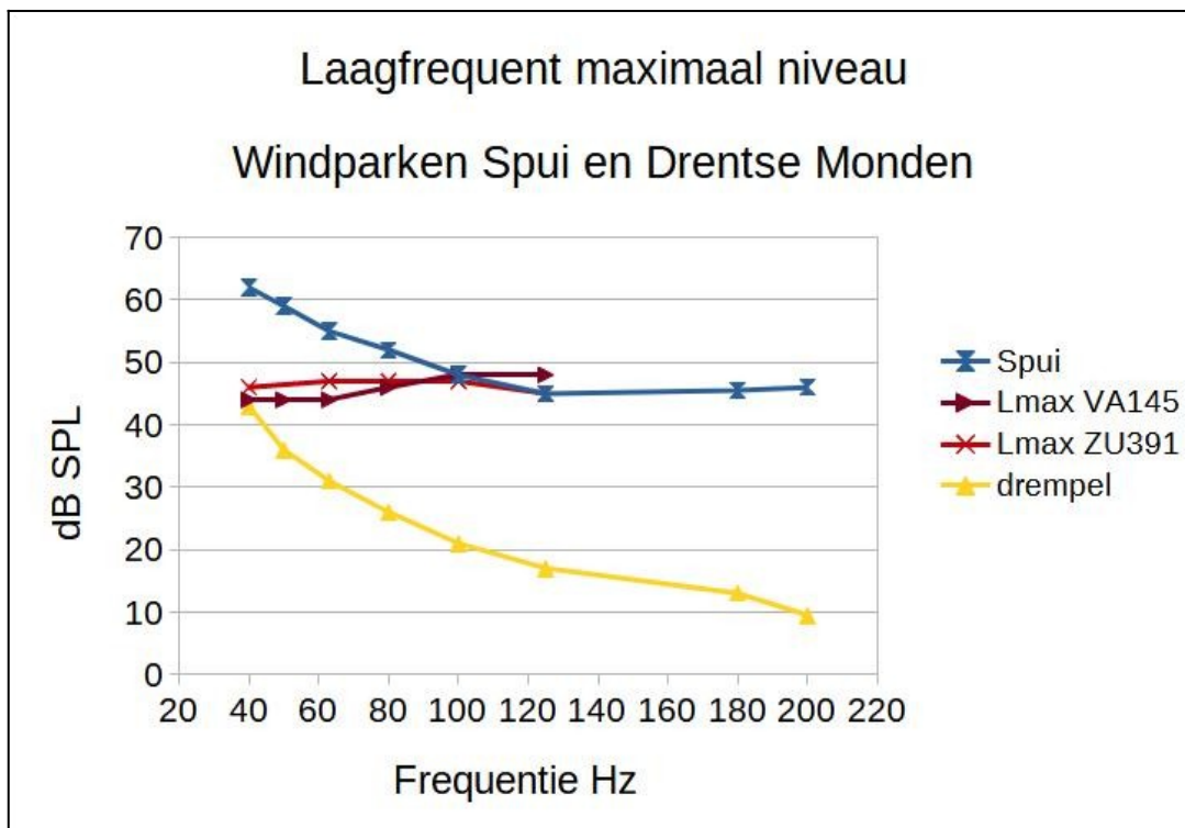
Figuur 5: Windparken Spui; Oostermoer en Drentse Monden. Maximaal laagfrequent geluidsniveau en gehoordrempel (ISO-28961- P10) Bron: 50,51
